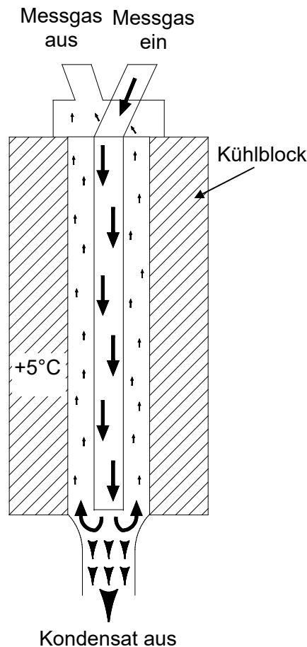
Abbildung 3 Funktionsschema des Wärmetauschers
