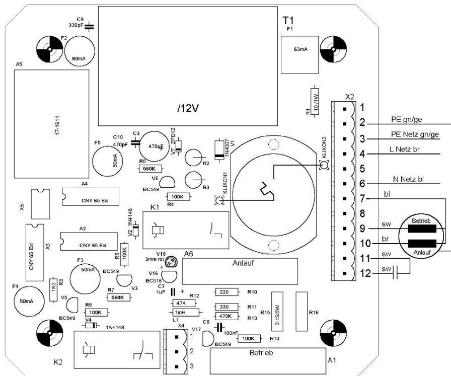
Abbildung 5 Aufbau der EC-EX-Regелеlektronik
