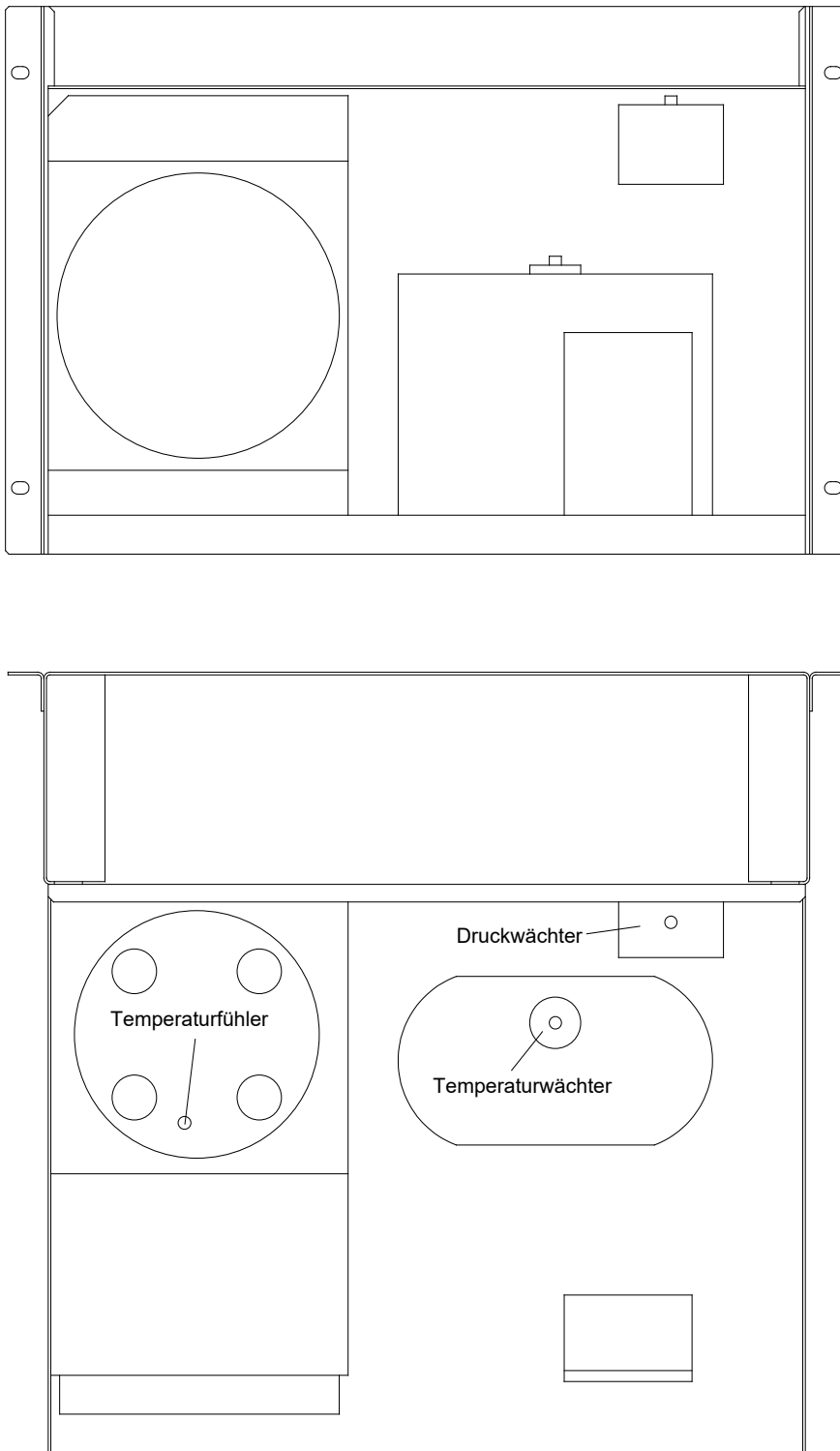
Abbildung 9 Schematische Darstellung EC-EX Kühler
