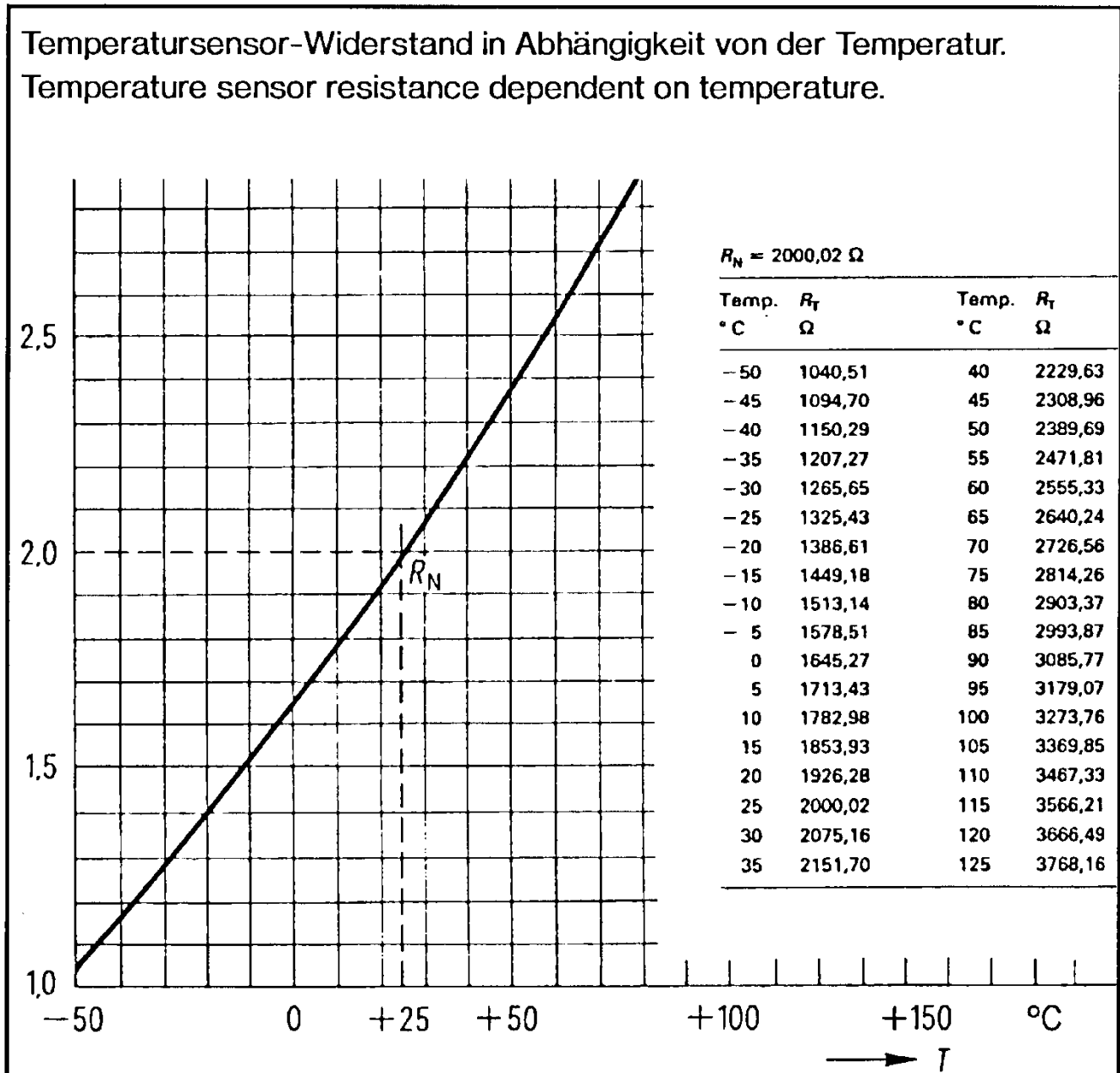
Abbildung 7 Temperatur-Widerstandscharakteristik des KTY-Temperatursensors
