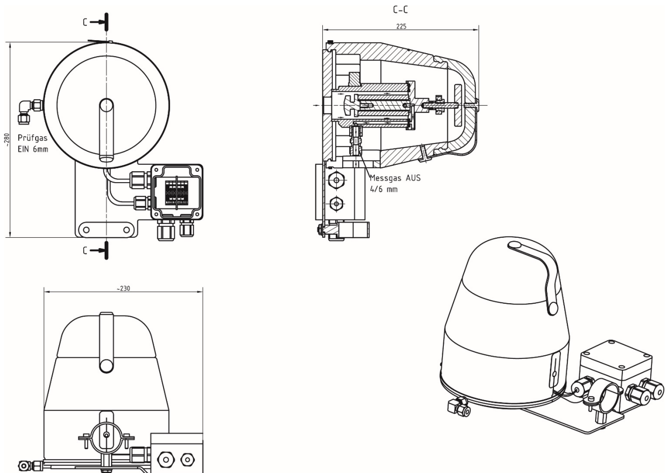
Abbildung 1 Abmessungen und Aufbau der SP180-H/MA
